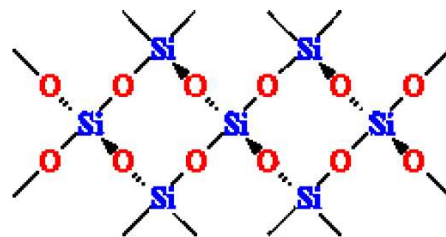
Kvartsin kiderakenne
