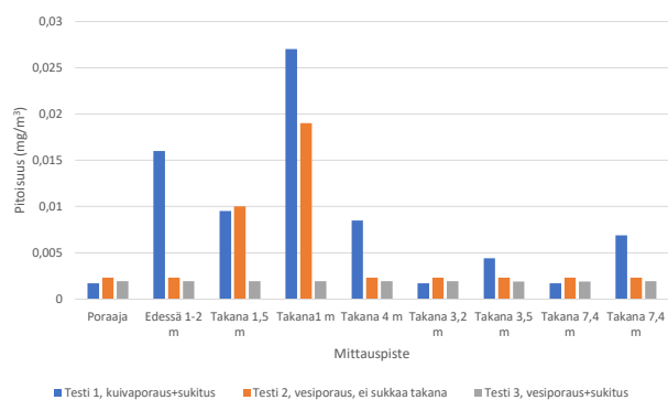
Kuvaaja 11. Alveolijakeisen kvartsin pitoisuuksia porausvaunun lähellä sekä poraajan altistuminen alveolijakeiselle kvartsille porattaessa vaihtoehdoilla polyntojuntatoimilla.
